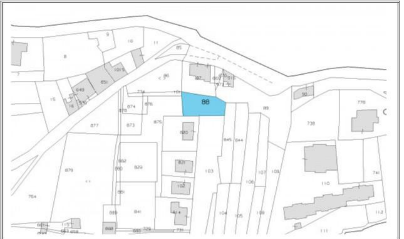
Planimetria
